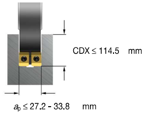
Tailor Made Dubbele tweezijdig snijdende schijffrees
