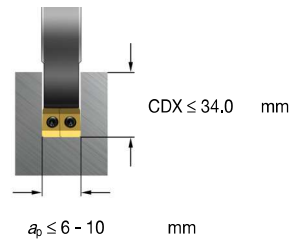
Volle groef vaste zitting
